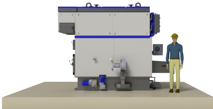
EKOMAT MR 650 kW
