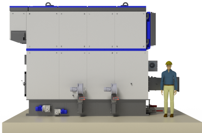
EKOMAT MR 2000 kW
